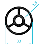
204.43 0,640 kg/m
