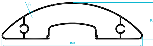
201.144 2,197 kg/m
