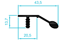
209.88 0,371 kg/m
