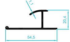
207.96 0,285 kg/m
