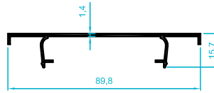
709.11 0,469 kg/m
