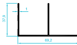
201.91 0,552 kg/m
