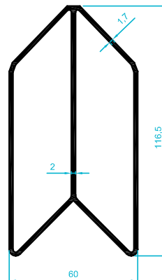
309.25 2,014 kg/m
