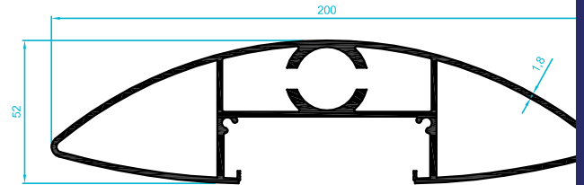
705.02 3,072 kg/m
