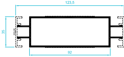
203.33 1,279 kg/m
