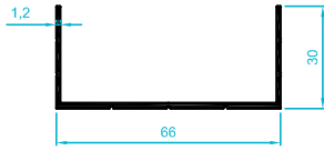
212.10 0,463 kg/m
