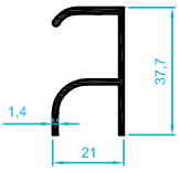
201.156 0,360 kg/m
