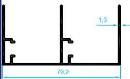
201.109 0,756 kg/m
