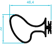
701.46 0,545 kg/m
