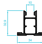
201.153 0,583 kg/m
