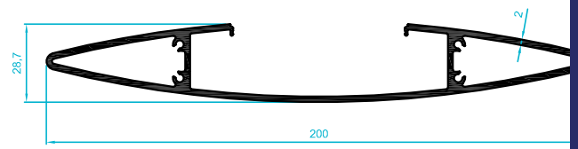
705.03 2,218 kg/m
