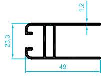
201.08 0,509 kg/m
