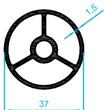
204.44 0,770 kg/m
