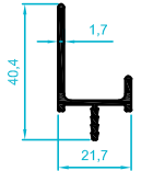
201.33 0,302 kg/m
