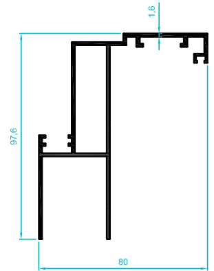
212.12 1,691 kg/m
