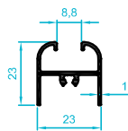
201.111 0,263 kg/m
