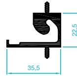
212.28 0,856 kg/m
