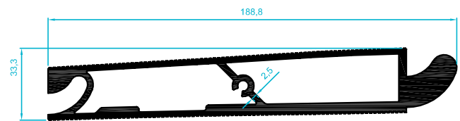
701.48 4,607 kg/m
