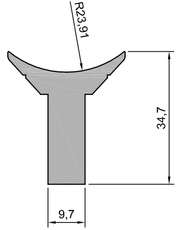
204.04 1,030 kg/m
