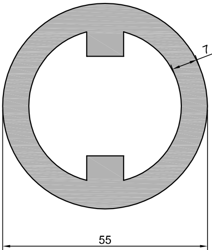
204.02 3,423 kg/m
