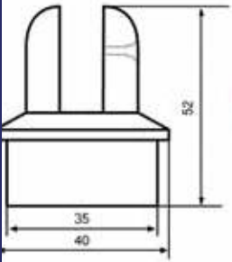
Ø 40'lik Boru Yarıkli Tapa
