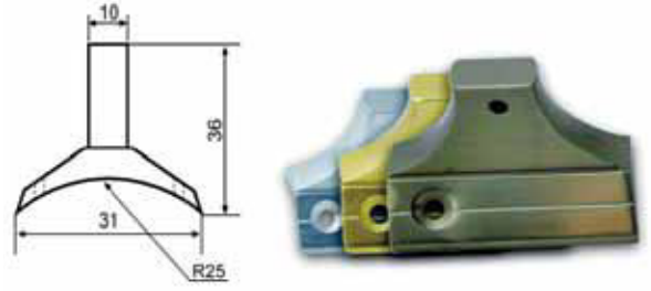
Ø 50'lık Boru Büyük Ay Bağlantı
