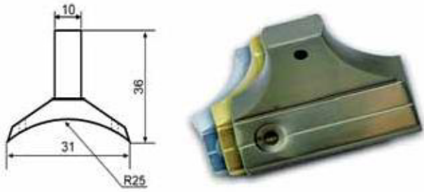
Ø 50'lık Boru Ay Bağlantı
