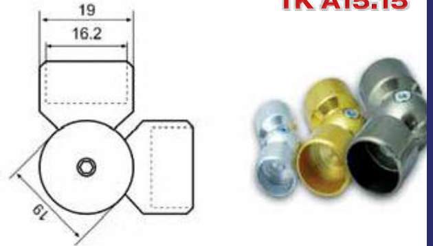
Ø 16'lik Ayarlı Küre Dirsek
