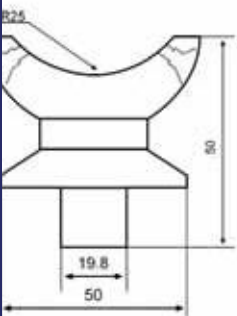
Ø 50x50 Dikme Dekorlu Sabit Mafsal
