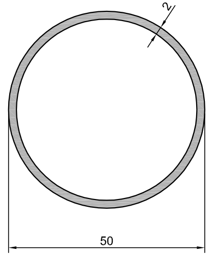
605.04 0,817 kg/m
