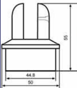
Ø 50'lik Boru Yarıkli Tapa
