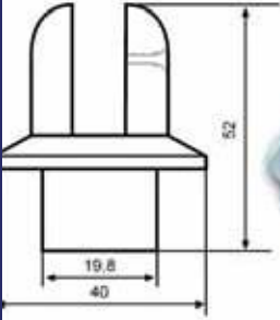
Ø 40'lik Dikme Yarıkli Tapa
