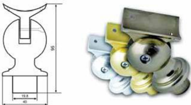
Ø 40'lık Topuz Mafsallı Takımı
