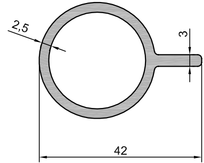
204.50 0,682 kg/m
