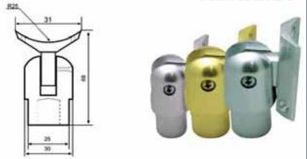
Ø 30'luk Boru Mafsallı Takımı
