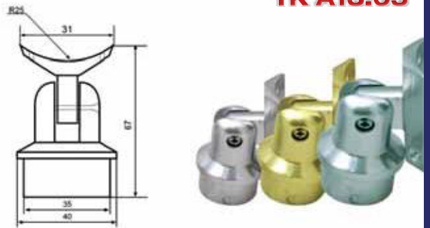
Ø 40'lık Boru Mafsallı Takımı
