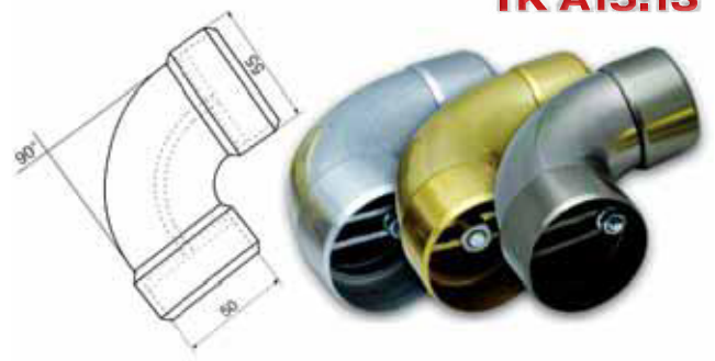
Ø 50'lik 1/4 Bilezikli Boş Dirsek
