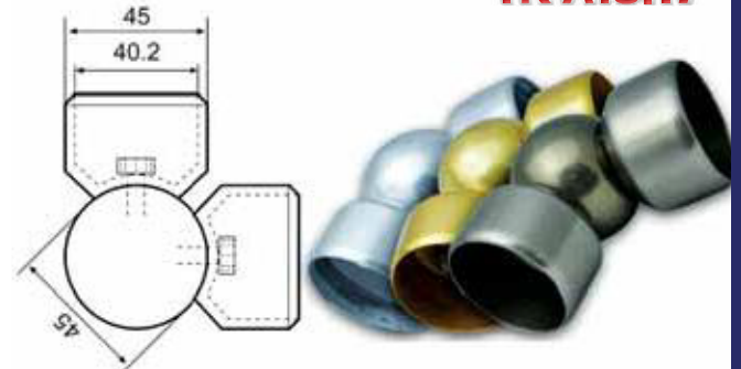
Ø 40'lik Ayarlı Küre Dirsek
