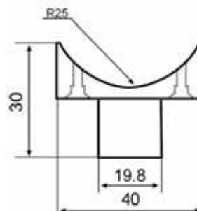
Ø 40x50 Dikme Ara Bağlantı
