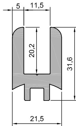
204.61 0,932 kg/m
