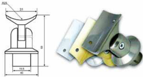
Ø 40'lık İkiz Dikme Mafsallı Takımı
