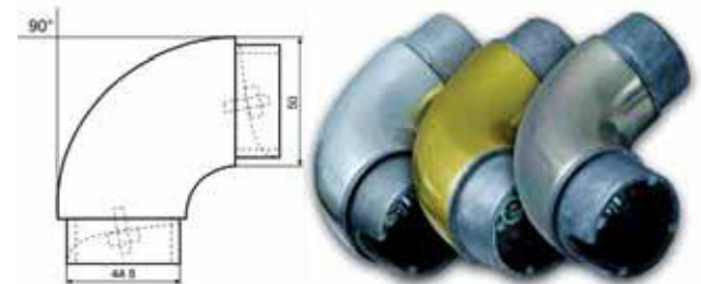
Ø 50'lik 1/4 Boş Dirsek
