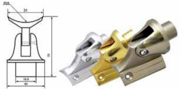
Ø 40'lık Dikme Dekorlu Mafsallı Takımı
