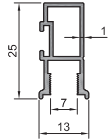
202.92 0,225 kg/m
