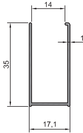
208.05 0,222 kg/m
