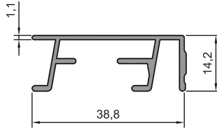
208.02 0,324 kg/m
