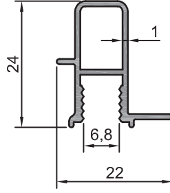
202.61 0,221 kg/m Fitilli Arka Kanat
