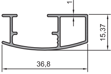
208.20 0,274 kg/m
