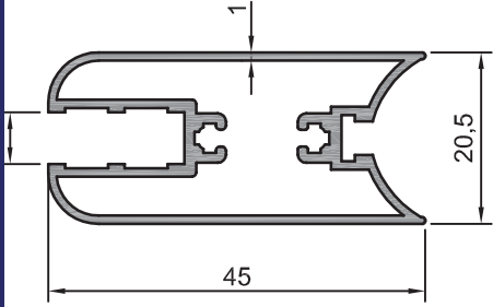
202.91 0,560 kg/m Menteşe Yatağı
