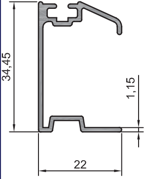
202.54 0,309 kg/m Dişi Ray
