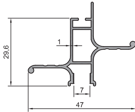
202.97 0,390 kg/m
