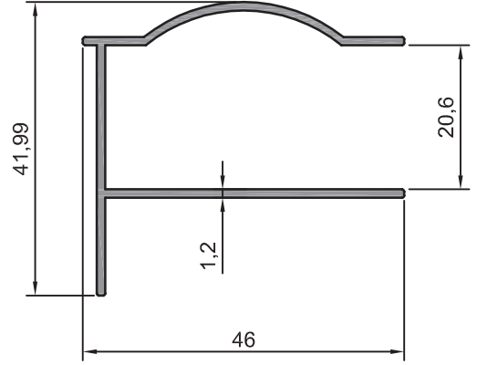
202.95 0,410 kg/m Duvar Dikmesi
