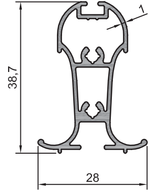
208.22 0,458 kg/m
