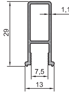
202.44 0,236 kg/m
