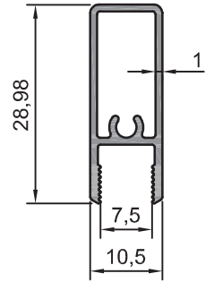
202.45 0,230 kg/m
