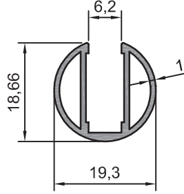
202.94 0,236 kg/m Kapı Menteşesi
