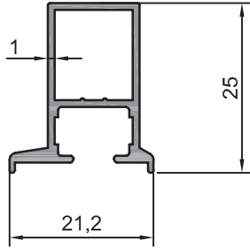
208.23 0,254 kg/m
