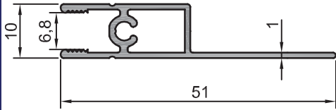
202.63 0,284 kg/m Fitilli Etek
