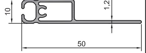
202.75 0,288 kg/m Silikonlu Etek
