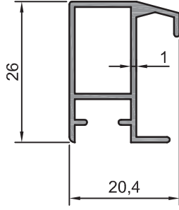
202.53 0,266 kg/m Erkek Ray
