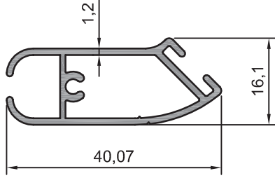
208.01 0,367 kg/m
