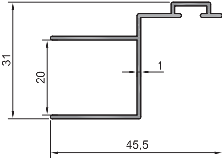
202.96 0,290 kg/m
