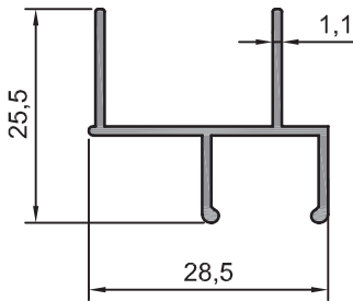
202.57 0,232 kg/m
