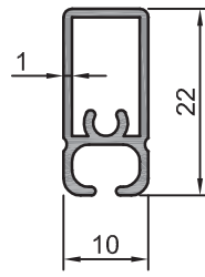
202.71 0,198 kg/m Silikonlu Panel Çıtası
