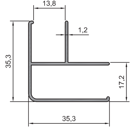
208.06 0,392 kg/m
