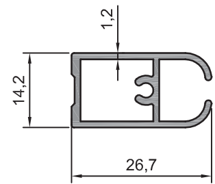
208.09 0,294 kg/m
