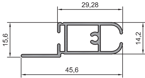
208.07 0,383 kg/m
