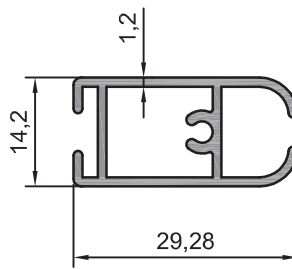
208.08 0,321 kg/m
