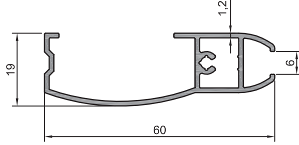
208.21 0,466 kg/m
