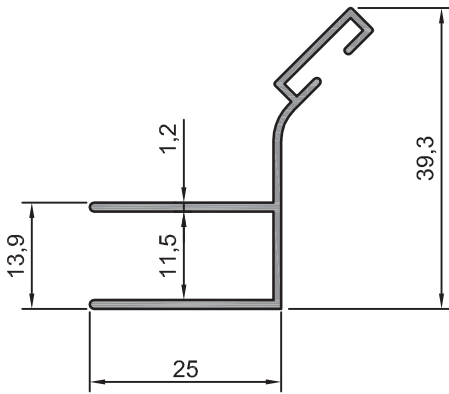
208.04 0,302 kg/m
