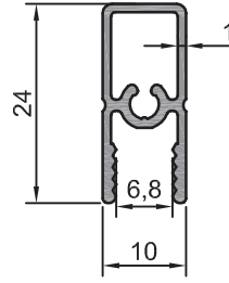
202.60 0,214 kg/m Fitilli Panel Çıtası
