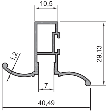
202.42 0,340 kg/m
