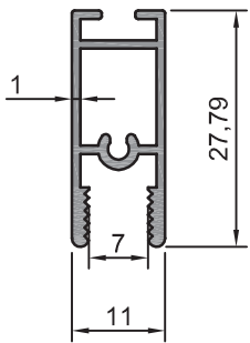
202.93 0,260 kg/m
