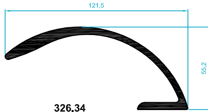
326.34 2,304 kg/m
