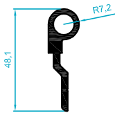
326.45 0,591 kg/m
